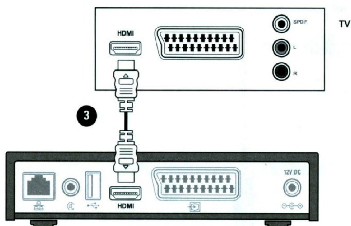
Obr. 4: Propojení set-top-boxu s televizorem pomocí HDMI kabelu (3).
