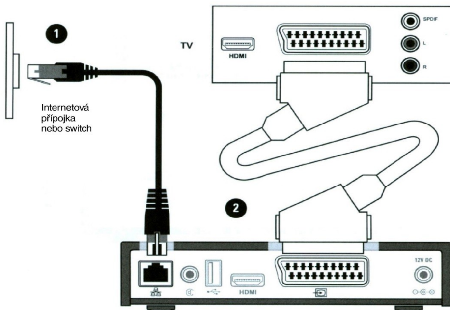
Obr. 3: Připojení set-top-boxu k síti M.NET (1) a k televizoru (2).
