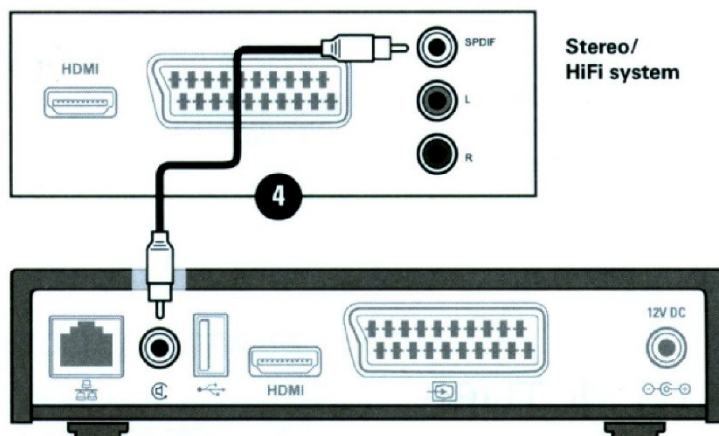
Obr. 5: Připojení zvuku kabelem SPDIF (4).
