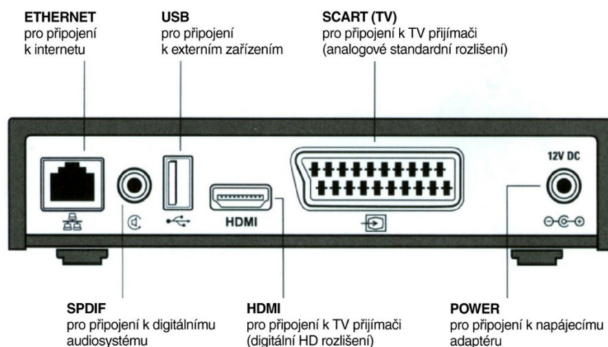
Obr. 2: Zadní panel set-top-boxu.
